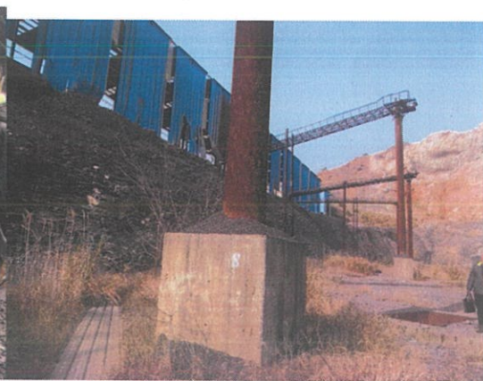
8#-1 皮带机及走道
