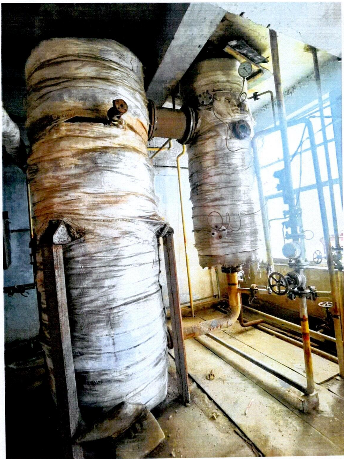
1、精制脱水塔一台 直径：800mm， 材质：304
